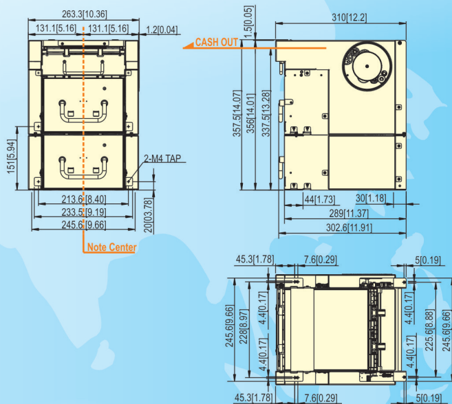
NDR2000
